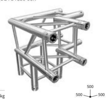
3-WEGE ECKE | 3-WAY CORNER C30 mit 95° Abgang rechts / with 95° joint right CODE F34C30-95R
