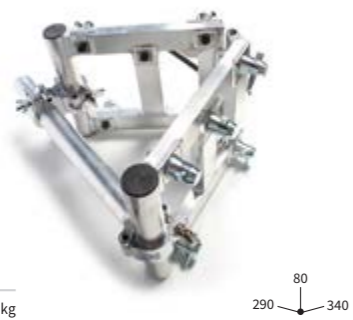
VARIABLE ECKE | CORNER 0-180° Der Winkel ist nur von ca. 20° bis 75° mit der mitgelieferten Stange arretierbar. CODE F34VC0-180
