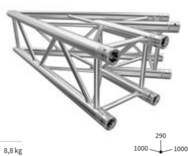
90° ECKE | CORNER C21 mit abgerundeten Ecken CODE F34C21-R500
