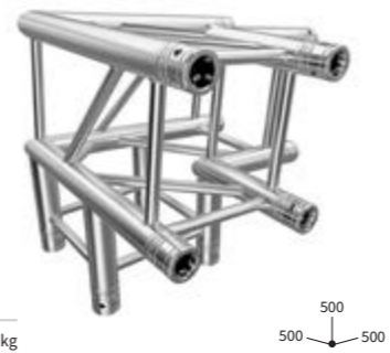
3-WEGE ECKE | 3-WAY CORNER C30 mit 85° Abgang links / with 85° joint left CODE F34C30-85L
